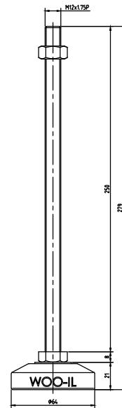
MFZ64-M12-250
