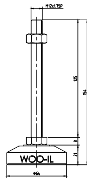
MFZ64-M12-125
