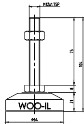
MFZ64-M12-75
