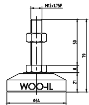
MFZ64-M12-50
