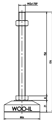
MFZ64-M12-150
