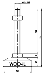
MFZ64-M12-100
