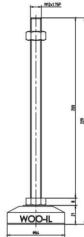
MFZ64-M12-200
