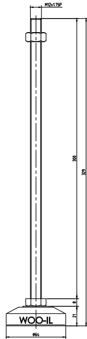
MFZ64-M12-300
