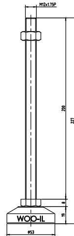
MFZ53-M12-200
