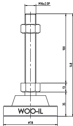
MFU78-M16-100
