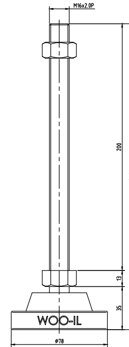
MFU78-M16-200
