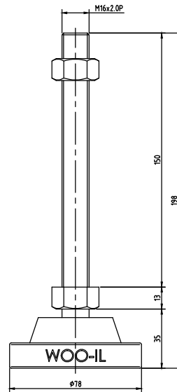
MFU78-M16-150
