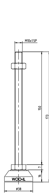
MFT38-M10-150
