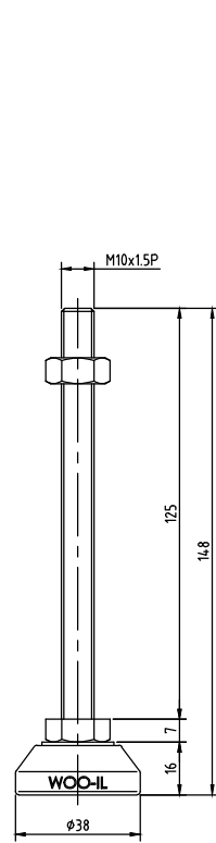
MFT38-M10-125
