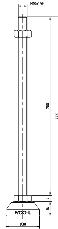
MFT38-M10-200
