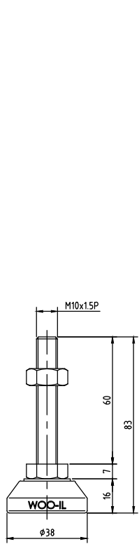
MFT38-M10-60
