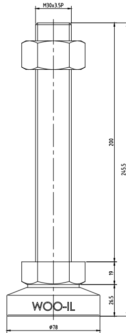
MFB78-M30-200
