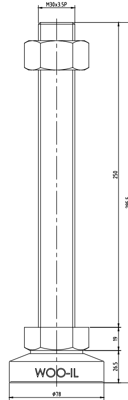
MFB78-M30-250
