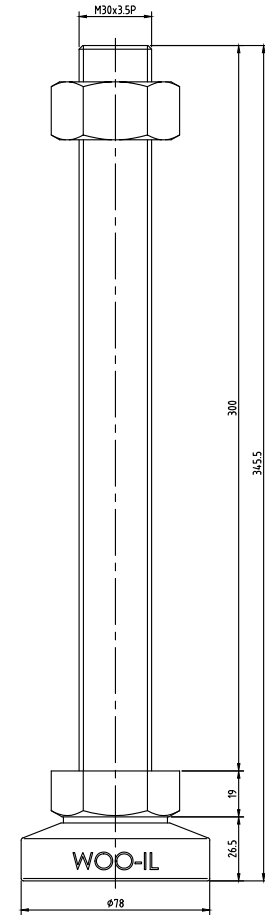
MFB78-M30-300
