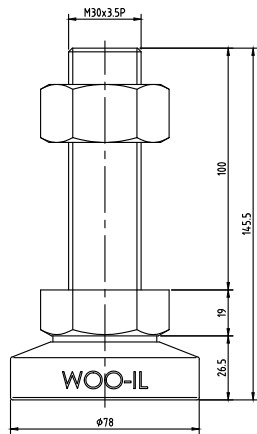
MFB78-M30-100
