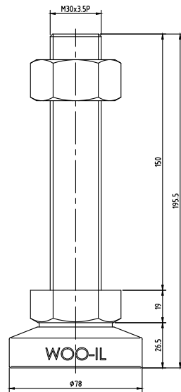
MFB78-M30-150
