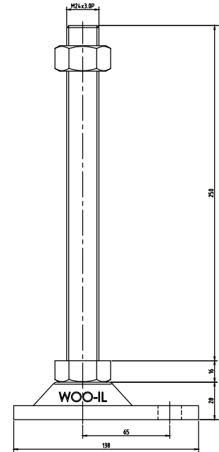
ARB103-M24-250
