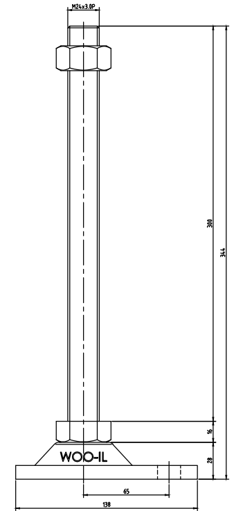
ARB103-M24-300
