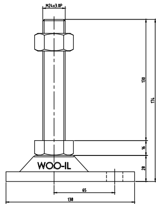
ARB103-M24-130
