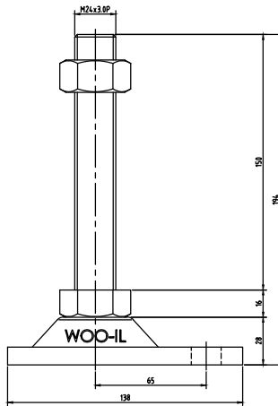
ARB103-M24-150
