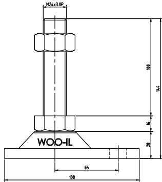
ARB103-M24-100
