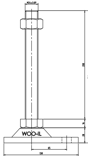
ARB103-M24-200
