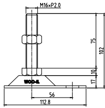
ABL76-M16-75
