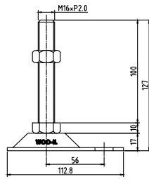
ABL76-M16-100
