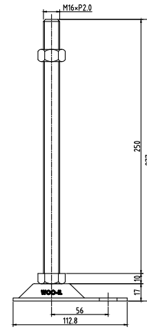
ABL76-M16-250
