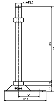
ABL76-M16-200
