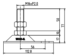
ABL76-M16-50
