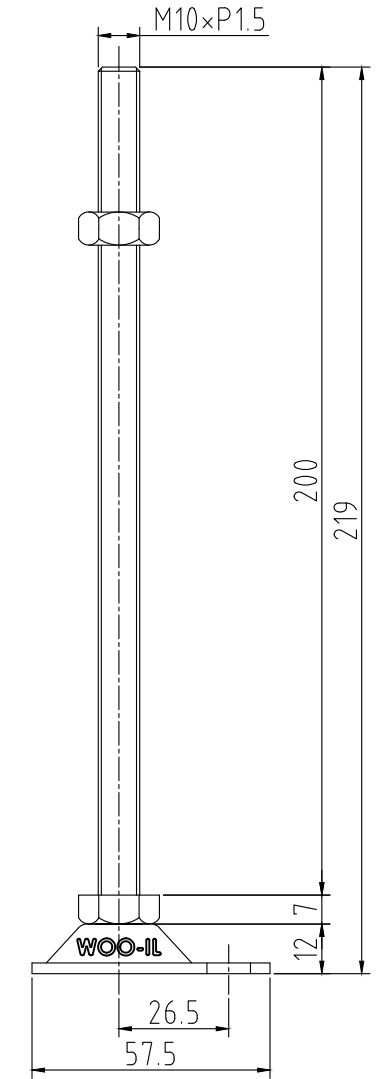
ABL42-M10-200
